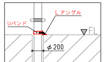
配管固定詳細 (S=1/30)
