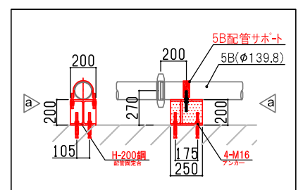
配管固定詳細 (S=1/30)
